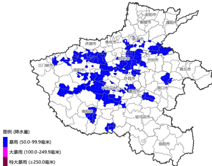
图 12025 年 8 月 6 日 9 时至 7 日 9 时暴雨分区预警
